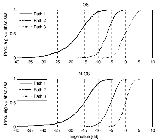
Fig. 6. Eigenvalue decomposition
